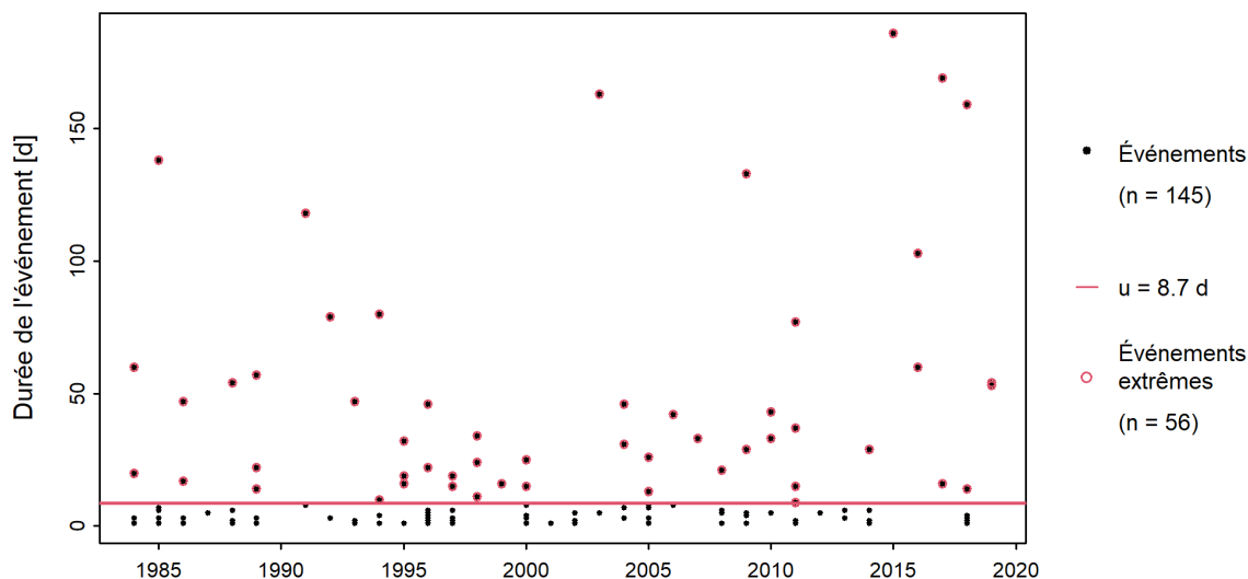
FIGURE 11 – Choix des événements extrêmes de durée d'ététiage utilisés pour la méthode POT
