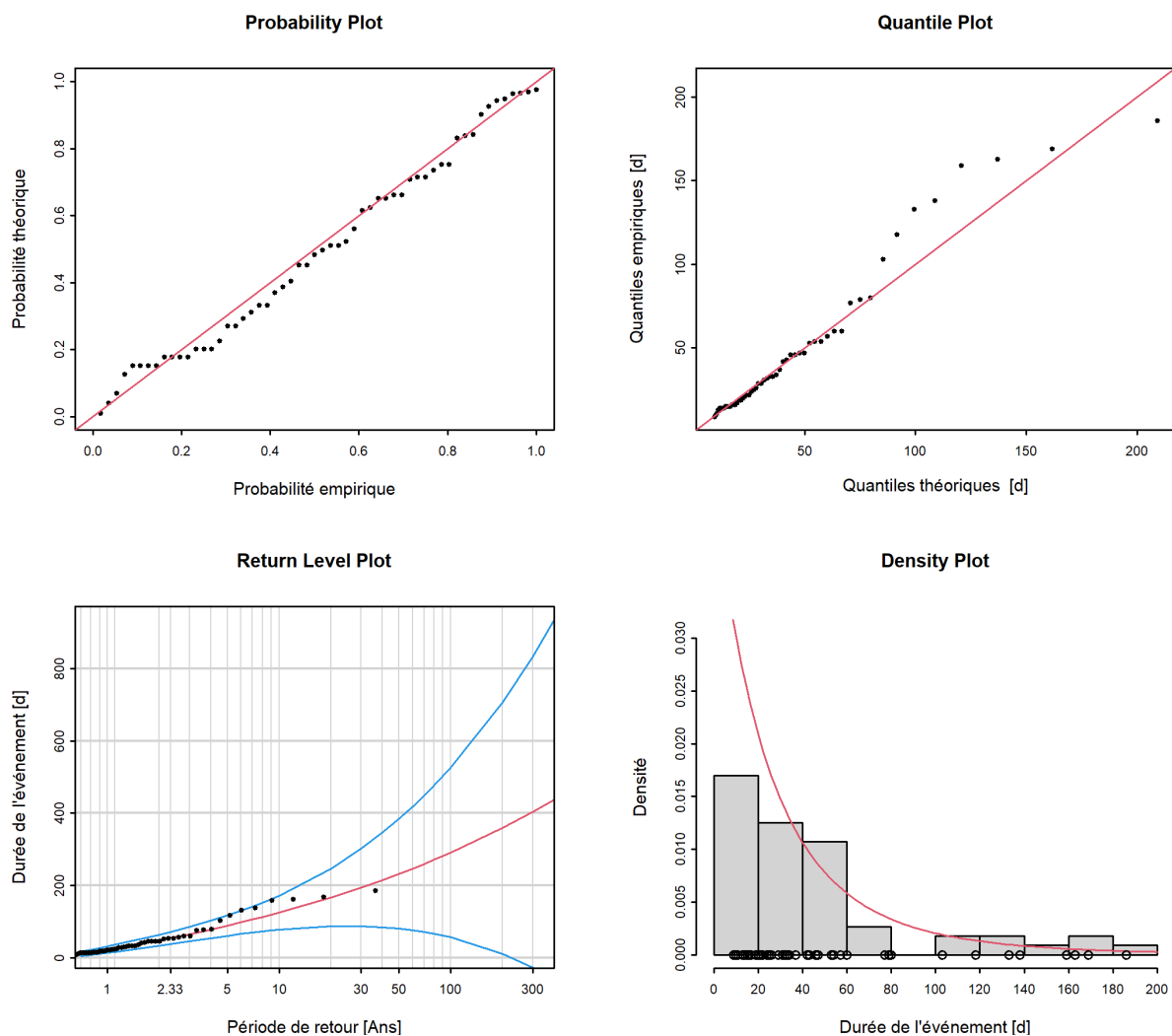
FIGURE 12 – Graphiques diagnostiques de la variante du modèle “ stat ” de la méthode POT (01.04.1984 - 31.03.2020)
