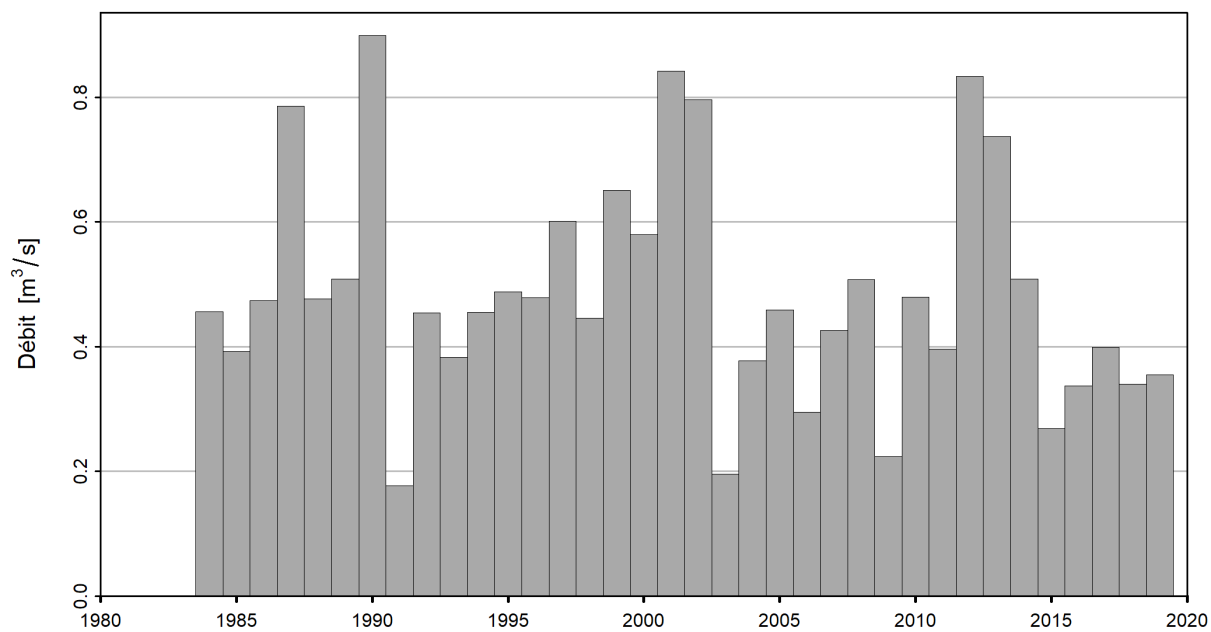
FIGURE 6 – Série temporelle de NM7Q [ \text{m}^3/\text{s} ] (01.04.1984 - 31.03.2020)
