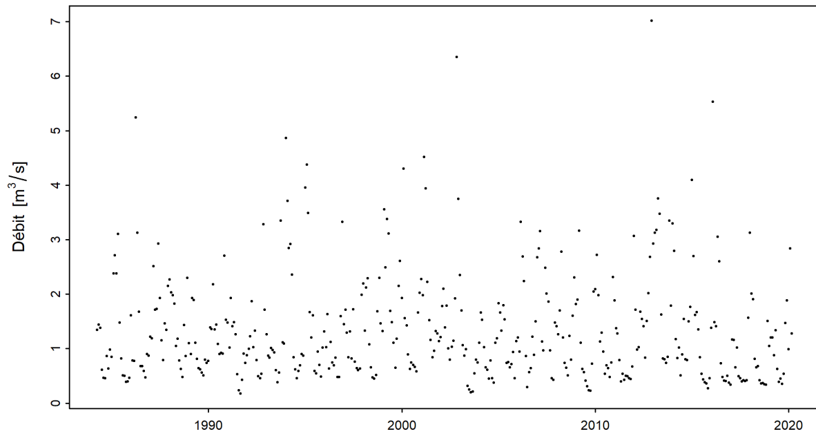
FIGURE 3 – Série temporelle du minimum mensuel de M7Q [ \text{m}^3/\text{s} ] (01.04.1984 - 31.03.2020)
