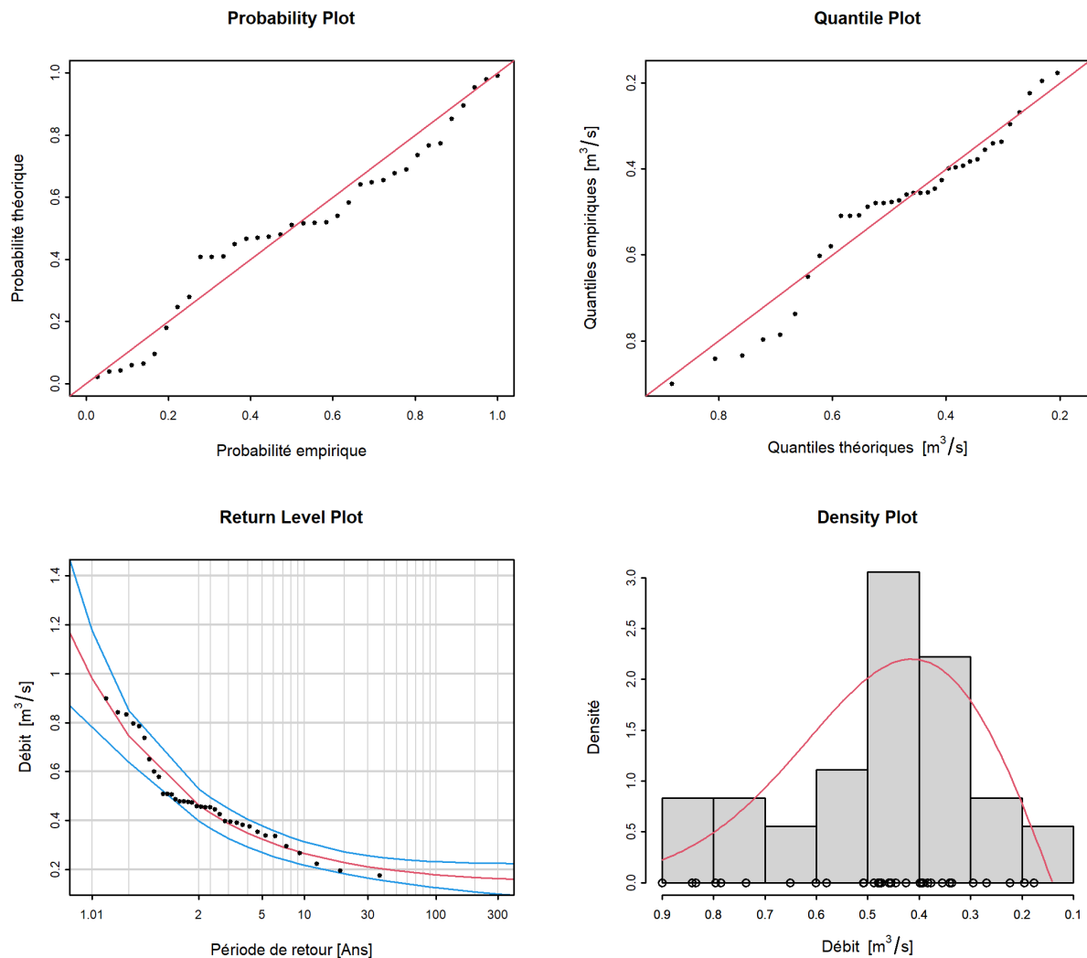
FIGURE 7 – Graphiques diagnostiques de la variante du modèle “ stat ” de la méthode BLOCK (01.04.1984 - 31.03.2020)
