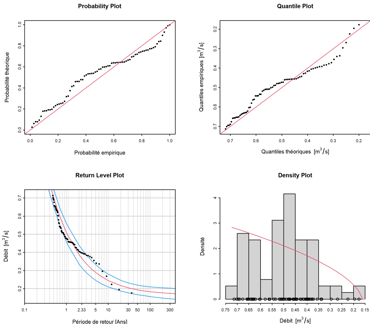
FIGURE 9 – Graphiques diagnostiques de la variante du modèle “ stat ” de la méthode POT (01.04.1984 - 31.03.2020)
