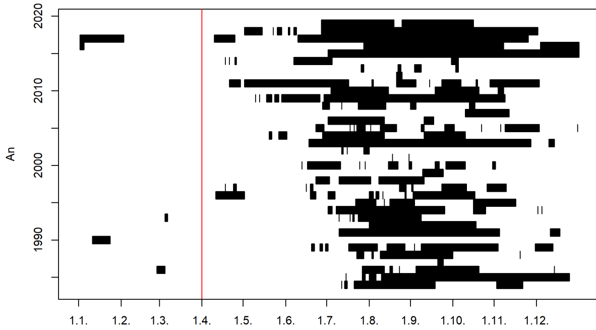
FIGURE 1 – Apparition temporelle des périodes d’étéage pendant l’année (01.04.1984 - 31.03.2020) et mois de début de l’année d’étéage (ligne rouge) 1
