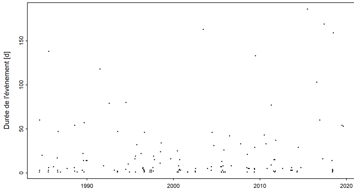
FIGURE 4 – Série temporelle des durées d'étéage [d] (01.04.1984 - 31.03.2020)
