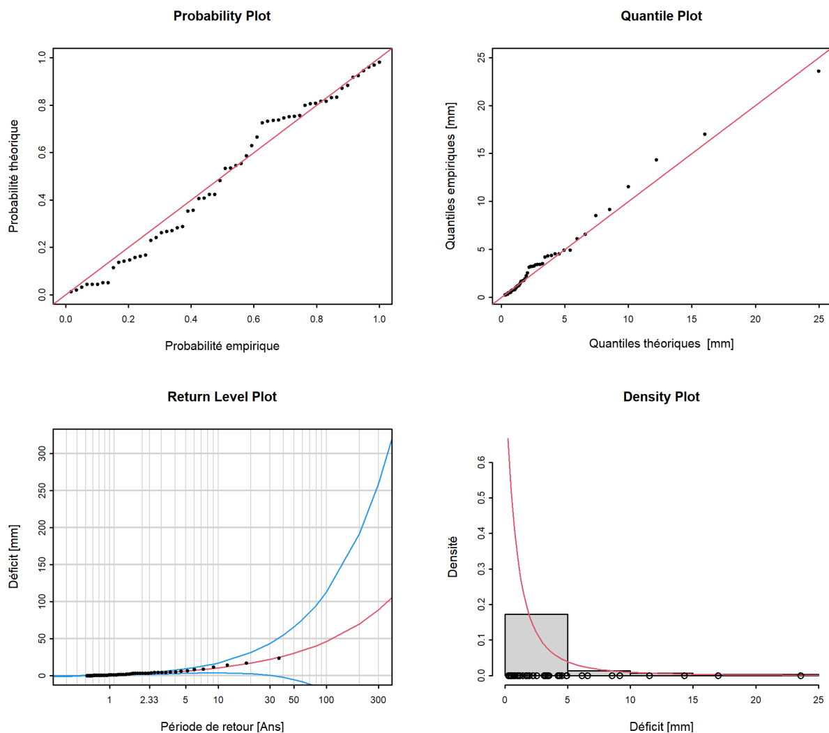
FIGURE 14 – Graphiques diagnostiques de la variante du modèle “ stat ” de la méthode POT (01.04.1984 - 31.03.2020)
