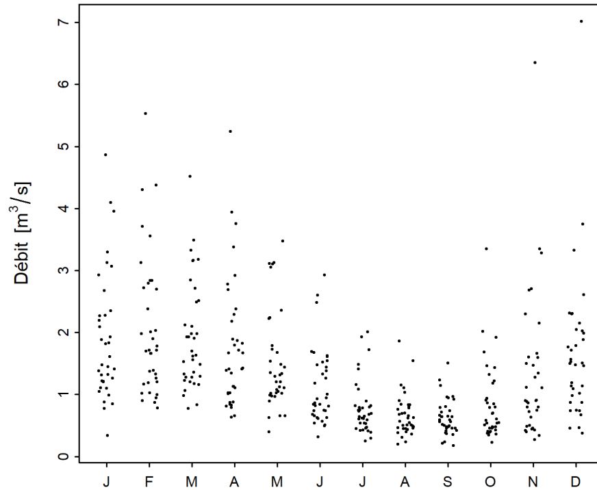
FIGURE 2 – Évolution saisonnière du minimum mensuel de M7Q [ \text{m}^3/\text{s} ] (01.04.1984 - 31.03.2020)
