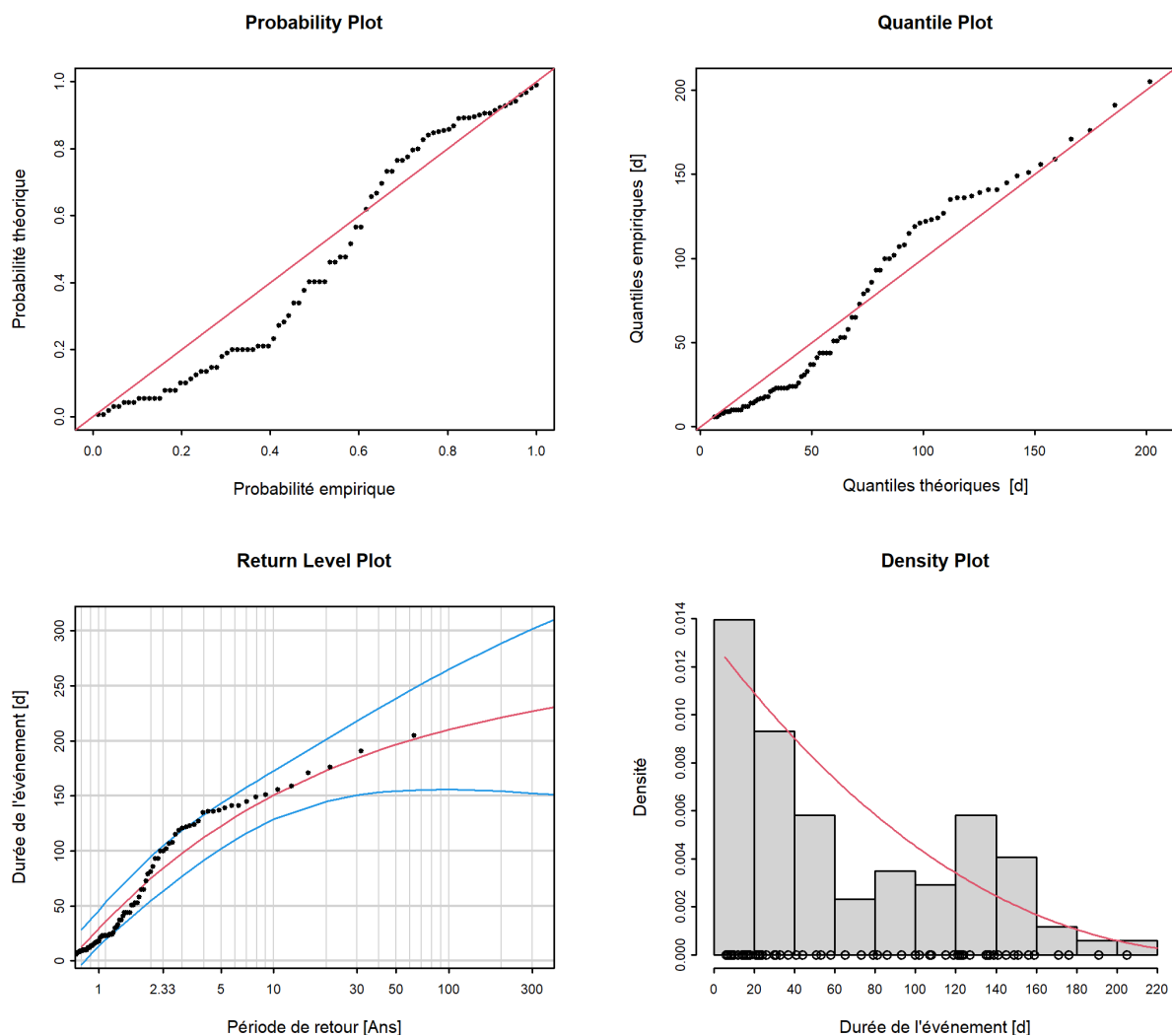
FIGURE 12 – Graphiques diagnostiques de la variante du modèle “ stat ” de la méthode POT (01.06.1957 - 31.05.2020)
