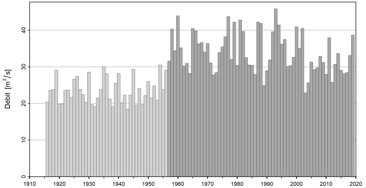
FIGURE 6 – Série temporelle de NM7Q [m³/s] (01.06.1916 - 31.05.2020), gris clair : NM7Q non utilisés, gris foncé : NM7Q utilisés
