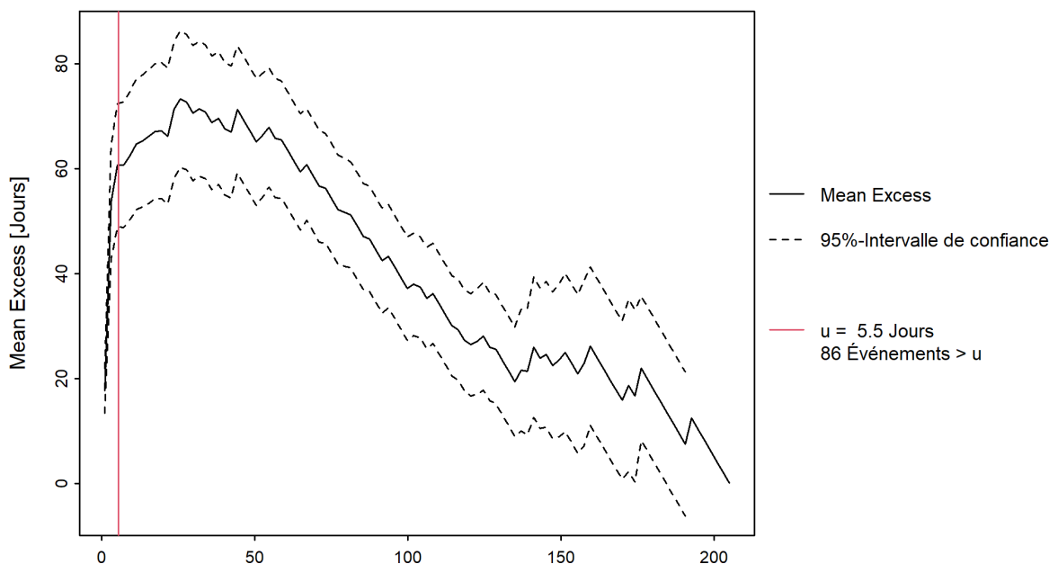
FIGURE 16 – “ mean residual life plot ” pour la durée d'étéiage
