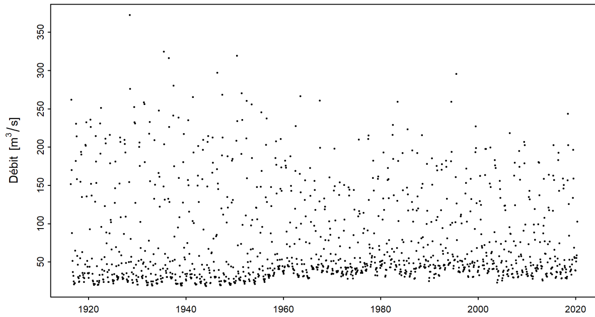
FIGURE 3 – Série temporelle du minimum mensuel de M7Q [ \text{m}^3/\text{s} ] (01.06.1916 - 31.05.2020)
