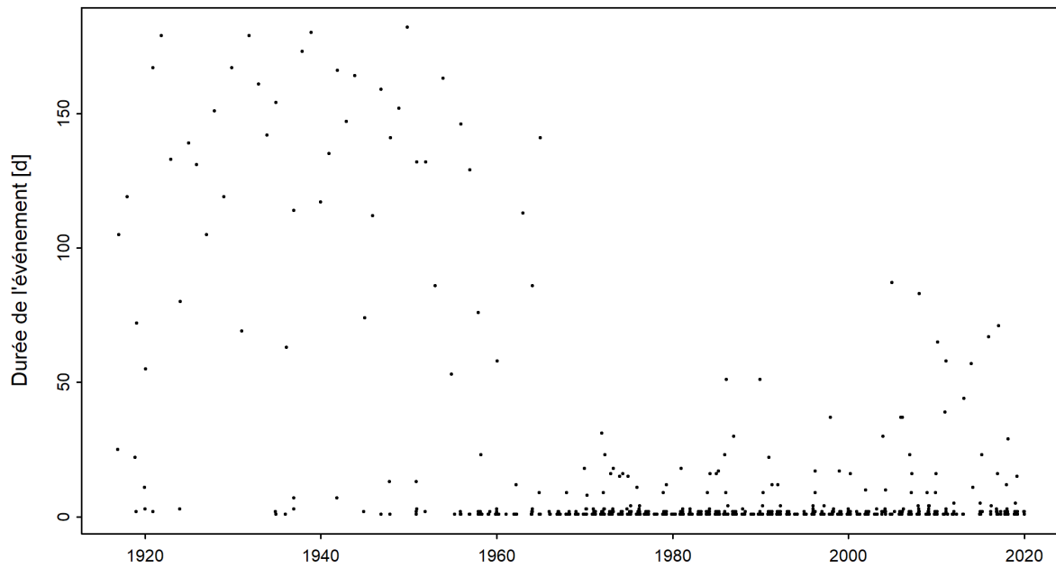
FIGURE 4 – Série temporelle des durées d'étéage [d] (01.06.1916 - 31.05.2020)
