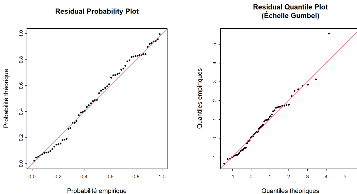
FIGURE 7 – Graphiques diagnostiques de la variante du modèle “ mujump2003 ” de la méthode BLOCK (01.06.1957 - 31.05.2020) Évaluation des graphiques diagnostiques (figure 7) :
