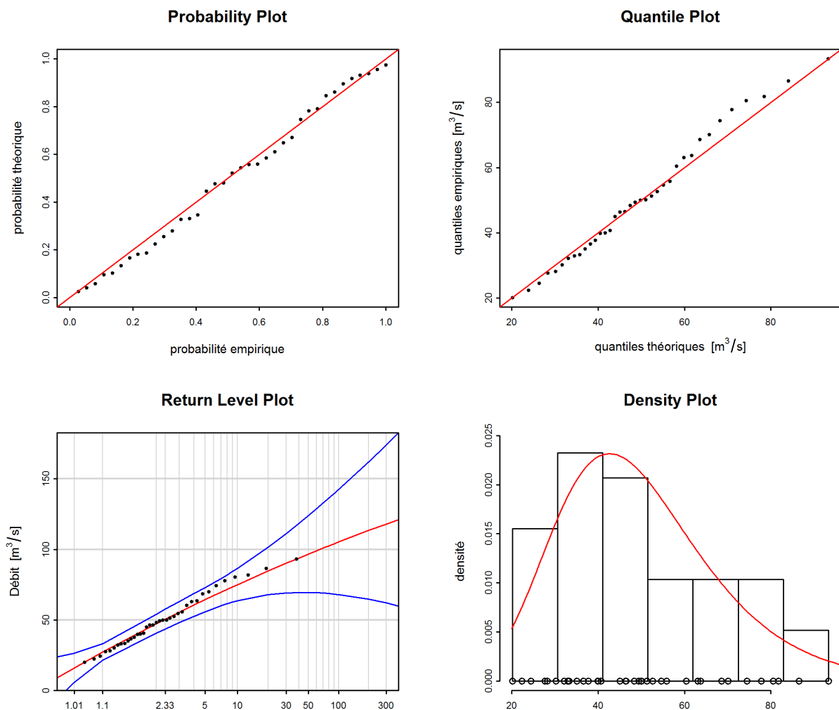
FIGURE 5 – Graphiques diagnostiques de la variante «stat» de la méthode BLOCK(1979-2015)
