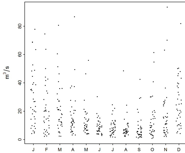
FIGURE 3 – Variations saisonnières des maxima mensuels [ \text{m}^3/\text{s} ] (01.01.1979 - 31.12.2015)
