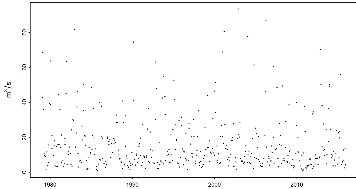
FIGURE 2 – Série chronologique des maxima mensuels [ \text{m}^3/\text{s} ] (01.01.1979 - 31.12.2015)
