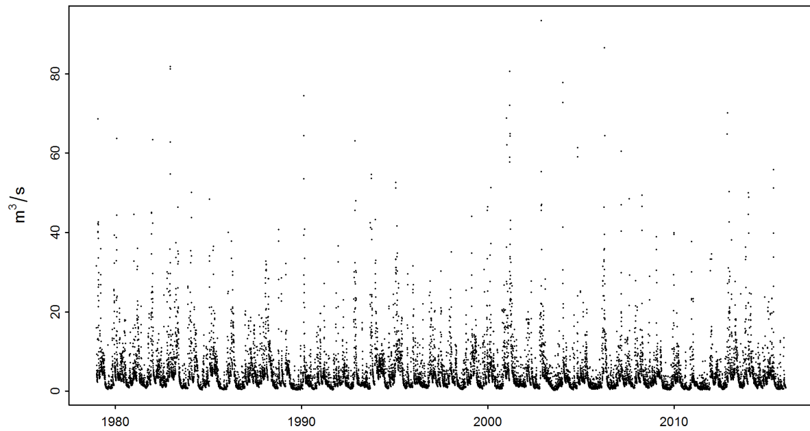
FIGURE 4 – Série chronologique des maxima journaliers [ \text{m}^3/\text{s} ] (01.01.1979 - 31.12.2015)
