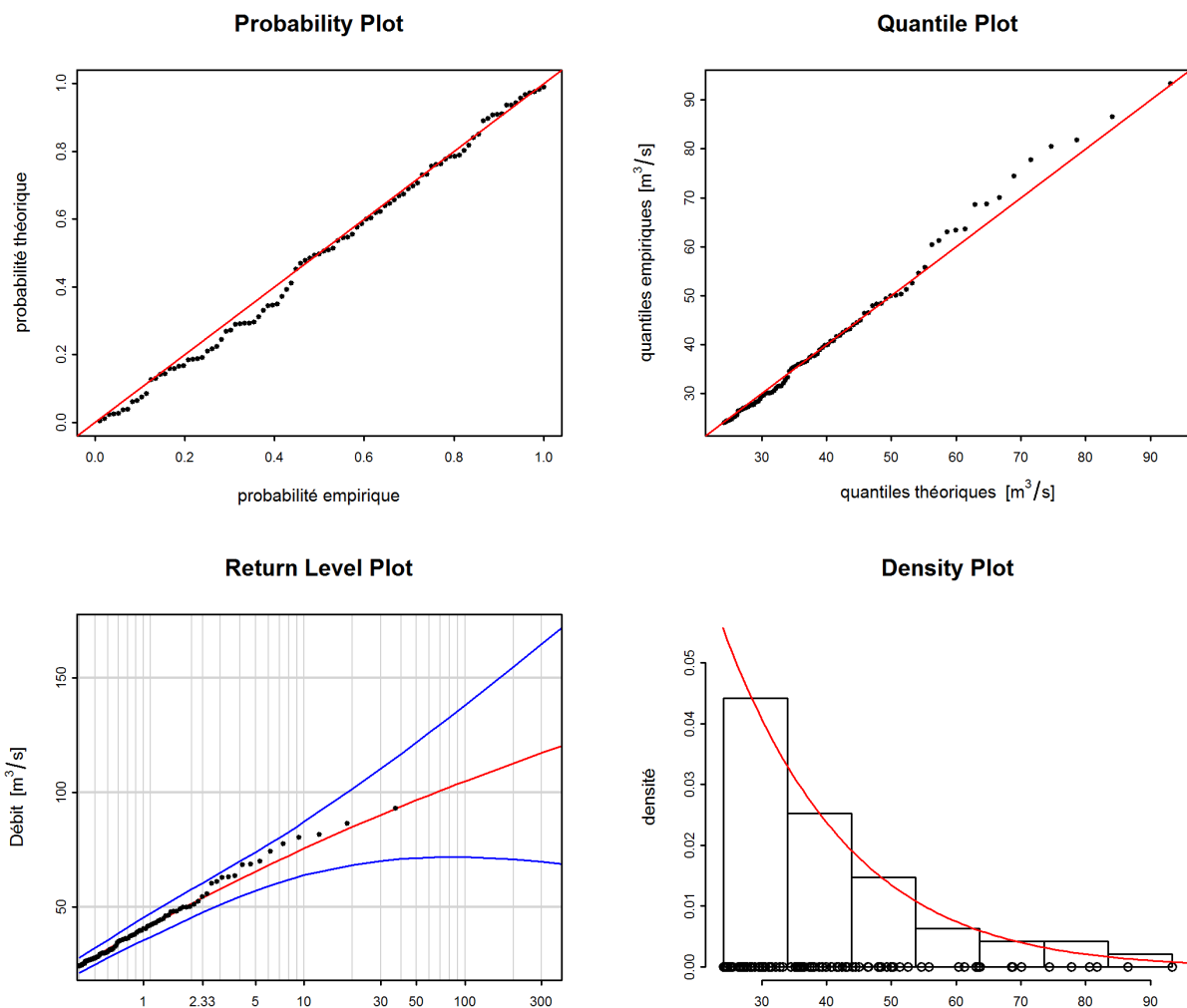
FIGURE 7 – Graphiques diagnostiques de la variante «stat» de la méthode POT (1979-2015)
