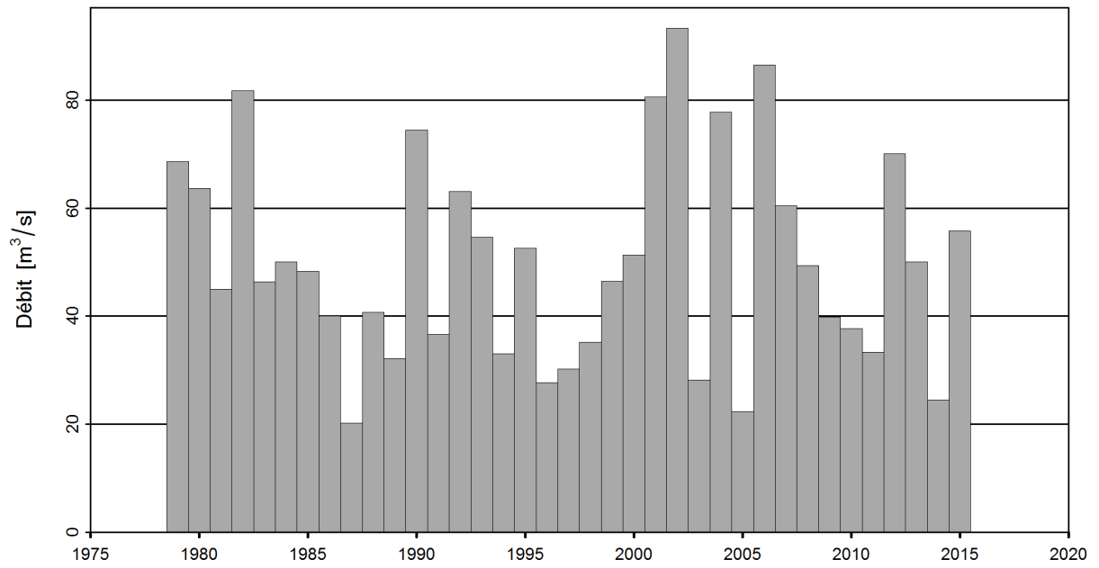
FIGURE 1 – Série chronologique des maxima annuels [ \text{m}^3/\text{s} ] (1979 - 2015, gris foncé : maxima annuels pris en compte)
