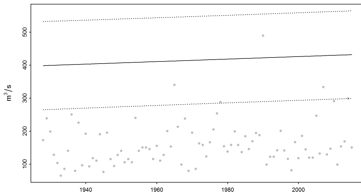
Abbildung 7: Veränderung der mit der Modellvariante „mul“ berechneten HQ 100 (durchgezogene Linien) und des 95%-Konfidenzintervalls (Deltamethode; gestrichelte Linien) über die Jahre 1928-2015
