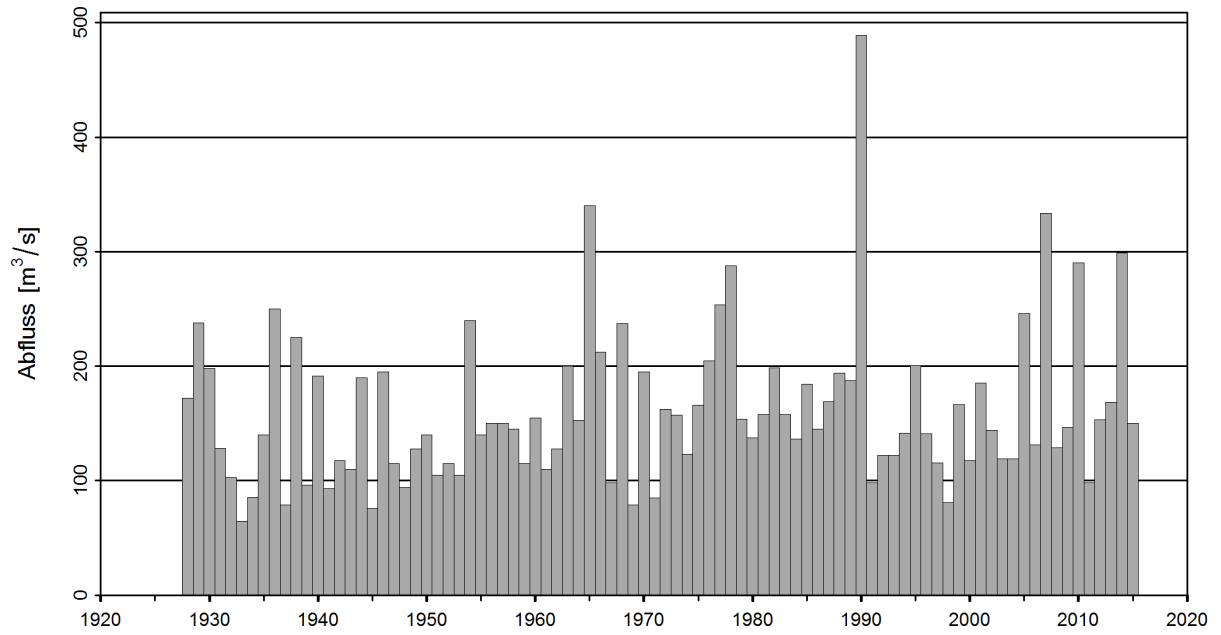
Abbildung 1: Zeitreihe der Jahresmaxima [ \text{m}^3/\text{s} ] (1928 - 2015, dunkelgrau: verwendete Jahresmaxima)
