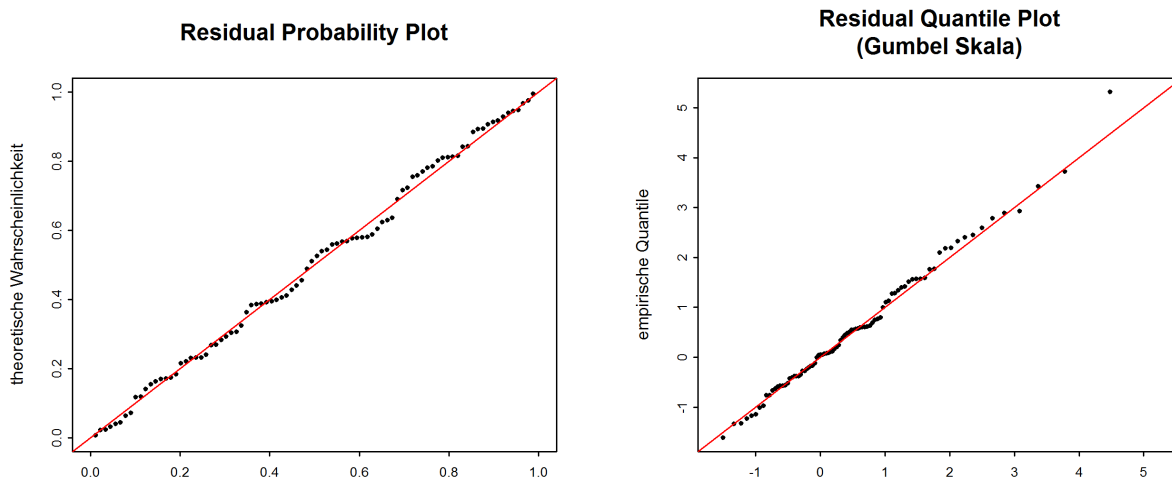
Abbildung 6: Diagnostikplots der Modellvariante „mul“ des BLOCK-Ansatzes (1928-2015)
