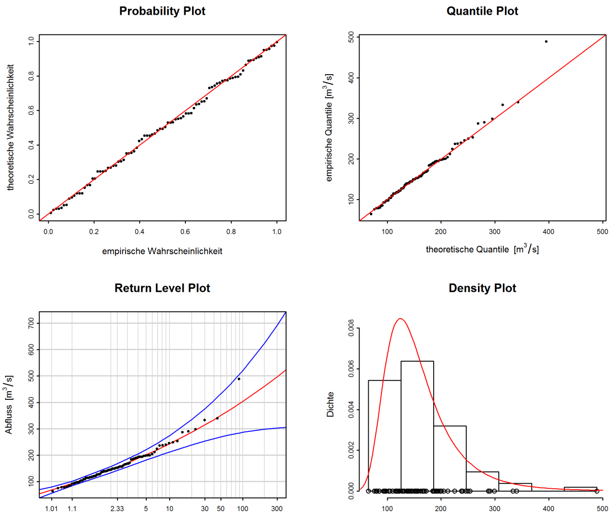
Abbildung 5: Diagnostikplots der Modellvariante „stat“ des BLOCK-Ansatzes (1928-2015)
