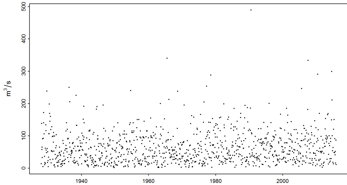
Abbildung 2: Zeitreihe der Monatsmaxima [ \text{m}^3/\text{s} ] (01.01.1928 - 31.12.2015)
