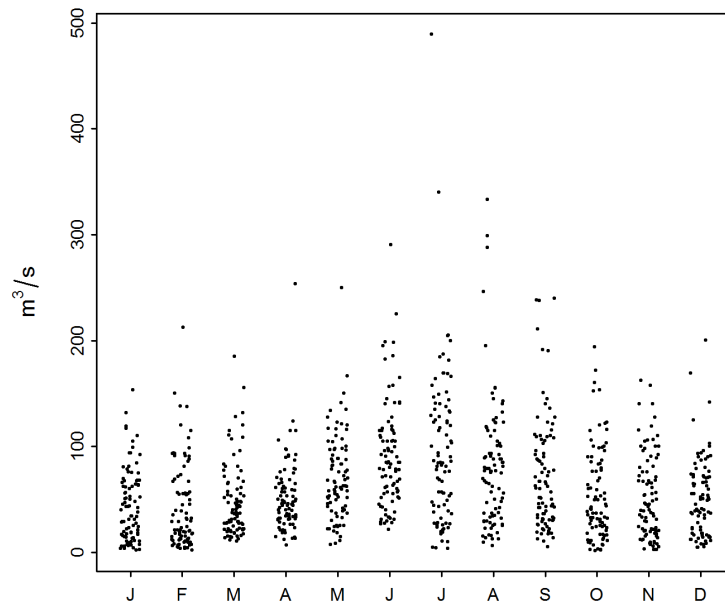
Abbildung 3: Saisonaler Verlauf der Monatsmaxima [ \text{m}^3/\text{s} ] (01.01.1928 - 31.12.2015)
